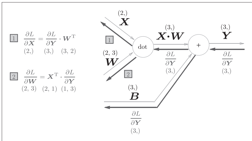
图 5-25 Affine 层的反向传播: 注意变量是 multidimensional array。反向传播时各个变量的下方标记了该变量的形状
